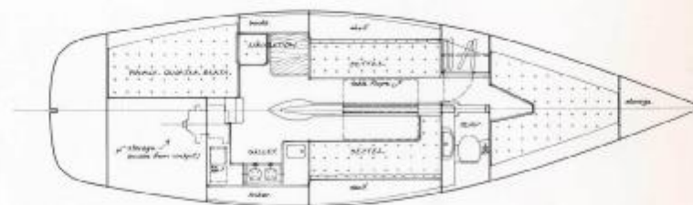
ARRANGEMENT.
