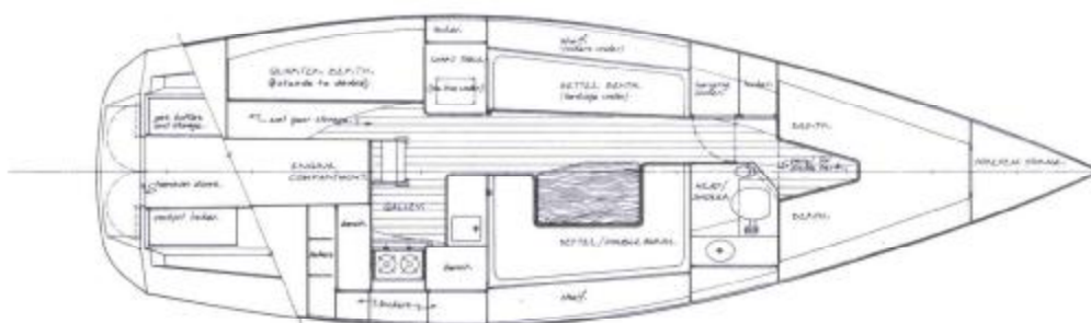
ARRANGEMENT.
